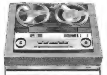
SABA HiFi-Stereo-Tonbandgerät 305 SH in eleganter Edelhölzarge. Frequenzumfang 40 – 18 000 Hz, Dynamik 50 dB, Bandgeschwindigkeiten 9,5/19 cm/s. Eingebauter Wiedergabeverstärker.
