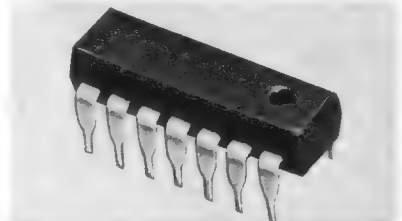
Integrierte Silizium-Plastik-Schaltkreise mit plastikvergossenem Gehäuse aus einem Stück haben gerade Anschlussdrähte zur Arbeitserleichterung für den Anwender.
