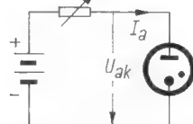
Bild 5. Schaltung zur Kennlinienaufnahme im Bereich oberhalb der Zündung der Glimmstrecke
