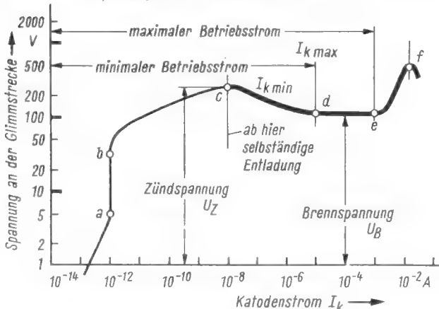
Bild 7. Gesamter Kennlinienbereich
