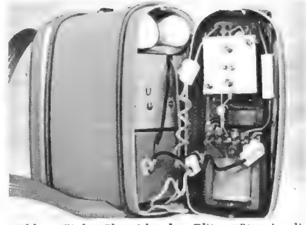
Bild 6. Einbauübersicht des Blitzgerätes in die Tragetasche
