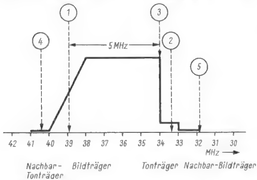
Bild 119. Theoretischer, idealer Verlauf der Durchlaßkurve eines Fernseh-Zwischenfrequenzverstärkers. Die in den Kreisen enthaltenen Zahlen mit Hinweispfeilen auf bestimmte Frequenzen entsprechen der Numerierung im Text
