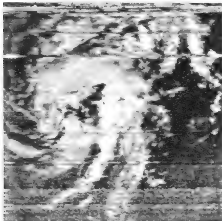
Bild 5. Tiefdruckgebiet über Europa, Essa 2, vom 4. 6. 66, 10.25 Uhr MEZ
