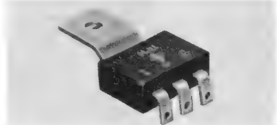
Durch den neuen TAB-PAC Leistungstransistor, der mit einer einzigen Schraube in verschiedenen Lagen montiert werden kann, wird das Befestigungsproblem elegant gelöst.
