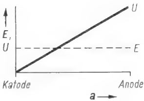
Bild 2. Spannungverteilung und Feldstärke in der Glimmröhre vor der Zündung
