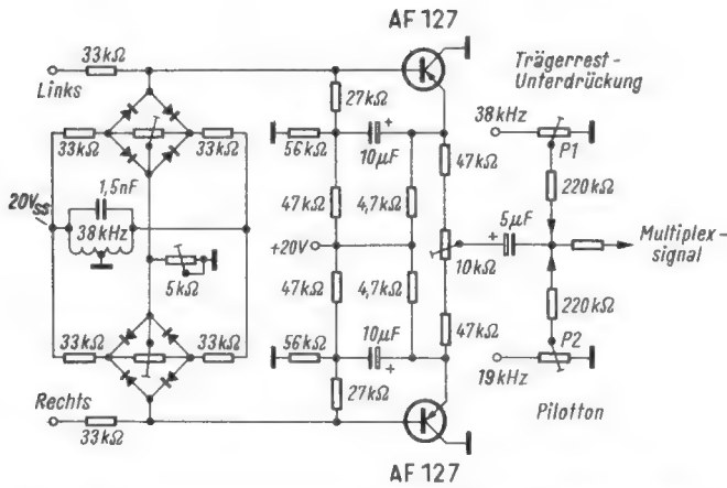
Bild 3. Der Zeitmultiplex-Modulator mit den beiden Diodenquartetten und die anschließende Addierstufe mit den beiden Transistoren AF 127
