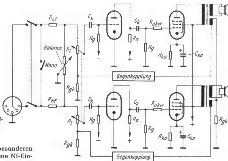
Rechts: Bild 29.12. Schema eines Zweikanal-Verstärkers für stereofone Wiedergabe
