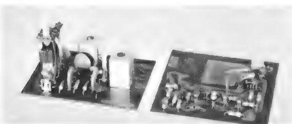
Vergleich des Versuchsaufbaus eines spulenlosen Ton-Zf-Teils für 250 kHz (rechts) mit einem in herkömmlicher Schaltungstechnik (links)
