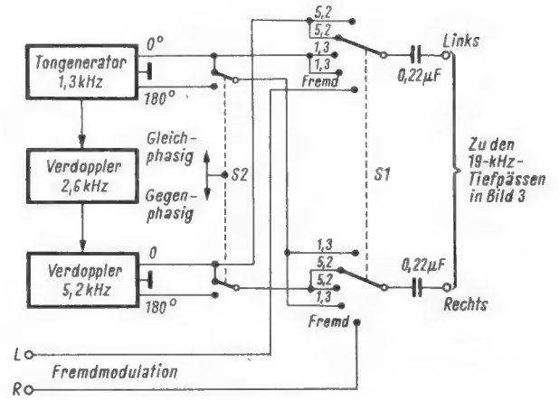
Bild 4. Die Modulationsmöglichkeiten des Stereocoders für Fremdmodulation oder die verschiedenen internen Modulationen
