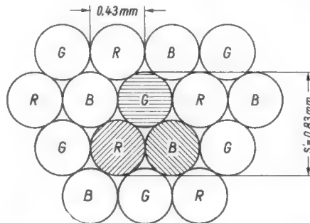
Bild 1. Anordnung und Größe der Leuchtpunkte für Blau, Grün und Rot bei einer Farbbildröhre
