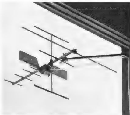
Die Kombinationsantenne Fesa F 208 wird mit Hilfe eines Kugelschalengelenkes am Fenesterräger befestigt. Die Länge der Antenne beträgt 69 cm, die des Trägers 54 cm
