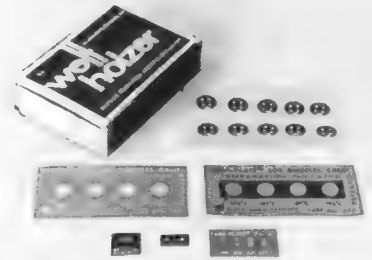
Die hellen Punkte auf den Temperaturplättchen färben sich bei Erreichen der aufgedruckten Temperaturwerte schwarz
