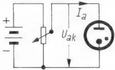
Bild 4. Schaltung zur Kennlinienaufnahme, wenn die Spannung an den Elektroden unterhalb der Zündspannung bleibt
