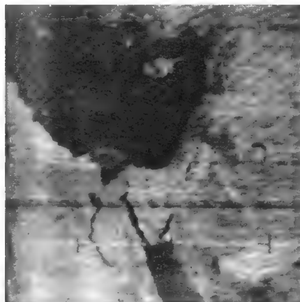
Bild 8. Nil-Delta und Rotes Meer, Nimbus 2, vom 9. 7. 66, 09.45 Uhr MEZ
