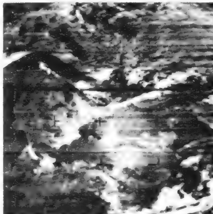
Bild 6. Spanien mit Mittelmeer, Nimbus 2, vom 26. 6. 66, 11.40 Uhr MEZ
