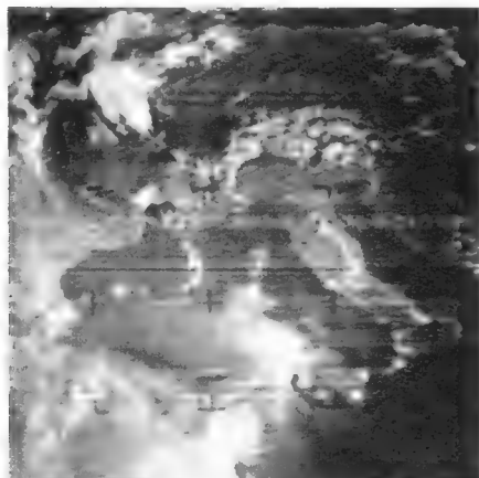
Bild 7. Mittelmeer mit Italien, Nimbus 2, vom 3. 7. 66, 11.25 Uhr MEZ
