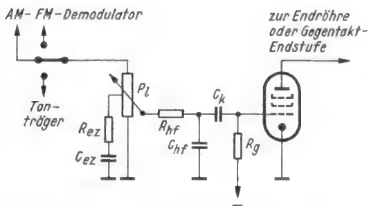
Bild 29.11. Umschalter am Nf-Verstärkereingang eines AM-FM-Empfängers
