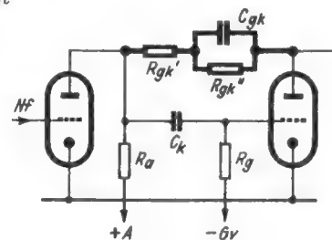
Rechts: Bild 30.4. Beispiel einer frequenzabhängigen Spannungs-Gegenkopplung über eine Stufe
